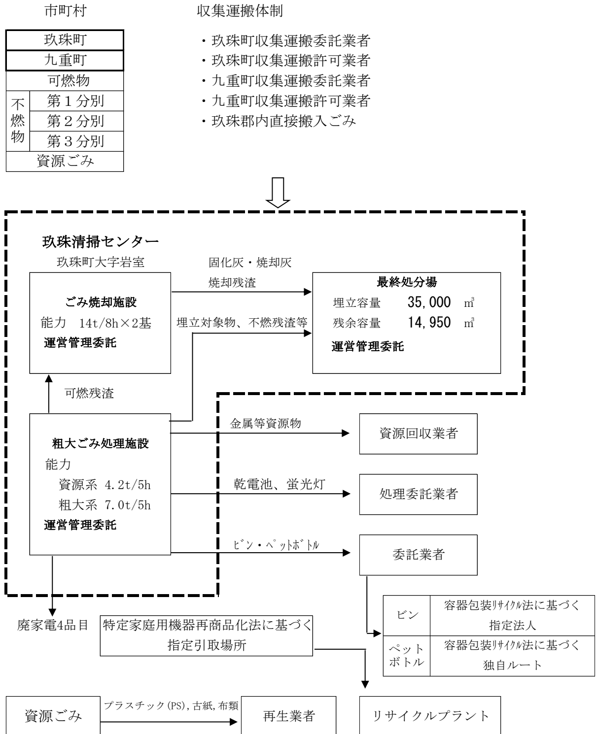
(1) ごみ処理計画フロー図
